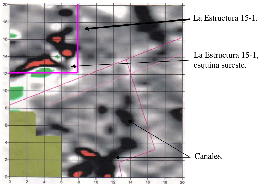
Fig. 6-3. Geoplot de la prospección gradiométrica realizado por Dr. David Monsees.
