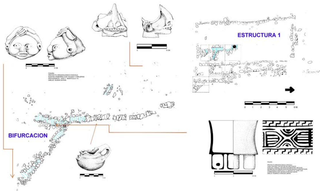
Fig. 6-2. Vista de Planta de la Estructura 15-1 incluyendo de vista de planta de los canales asociados y artefactos recuperados, PACH 2004.
