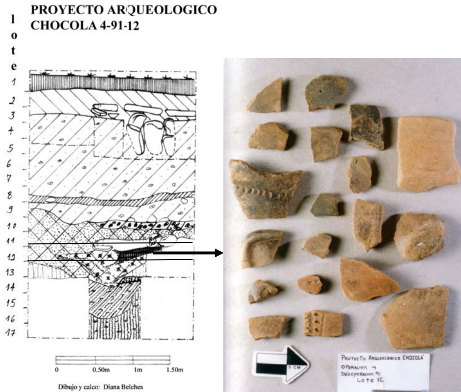
Fig. 6-36. Ejemplos de perfiles de la cerámica recuperada en dos pozos dentro de la Estructura 15-1, con fechamiento por radiocarbóno.
