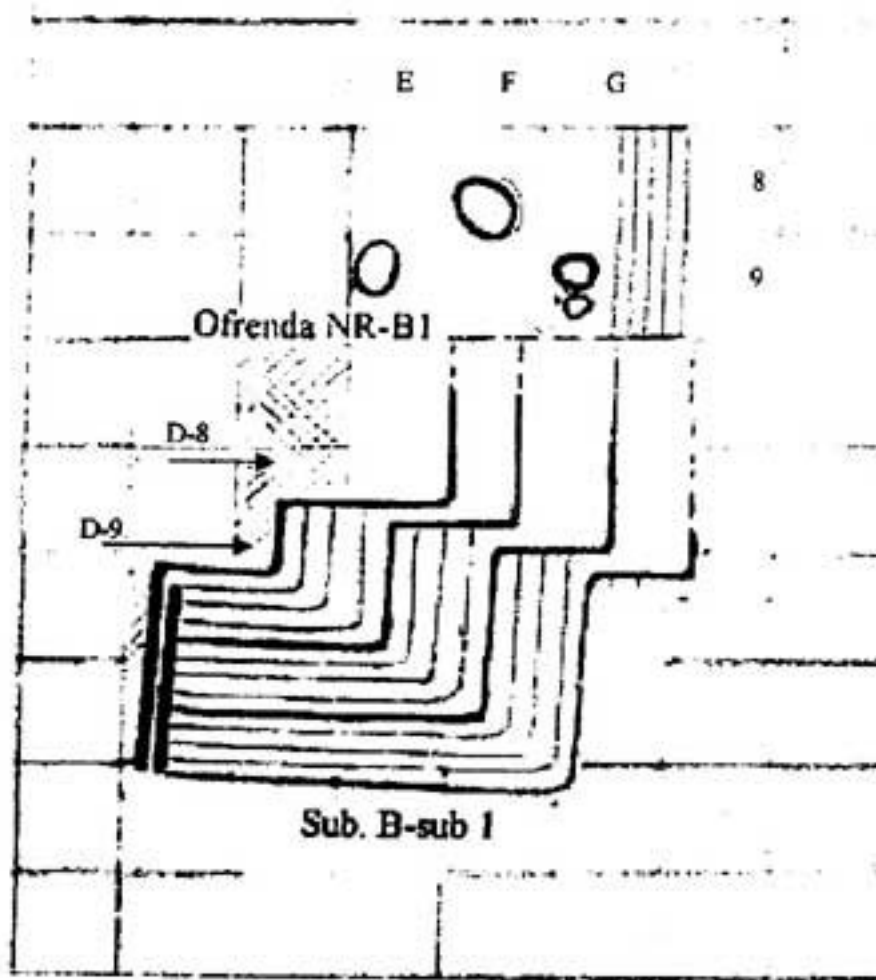
Figura 8a. Detalle de excavación de pozos.
