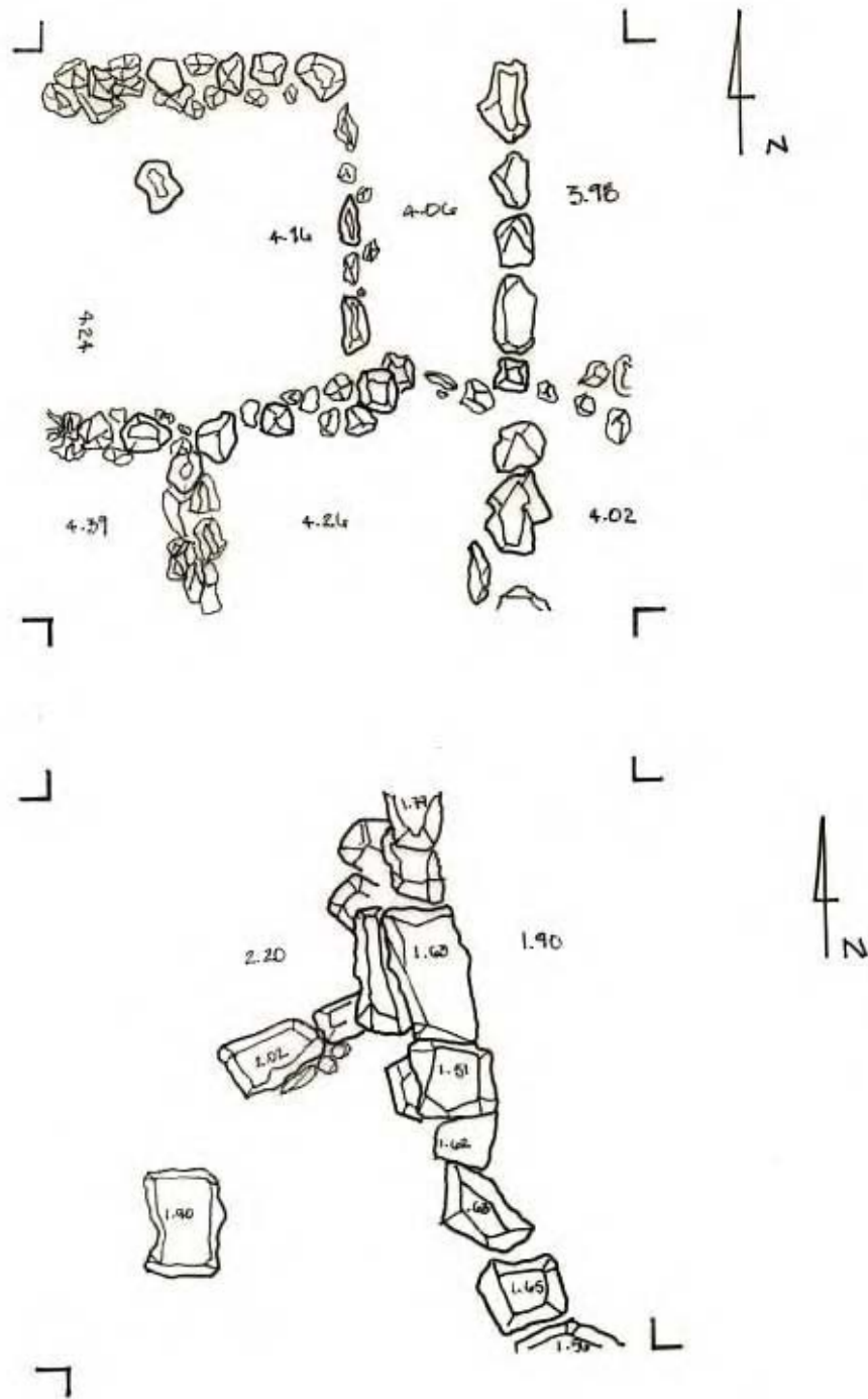
Figura 19c. Subestructura B-sub 2. Planta de remodelaciones.
