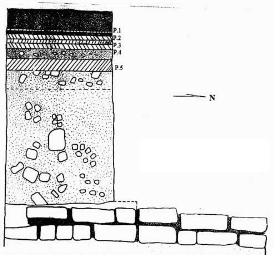
Figura 12b. Estructura B-sub 1, registro en sector de escalinata.
