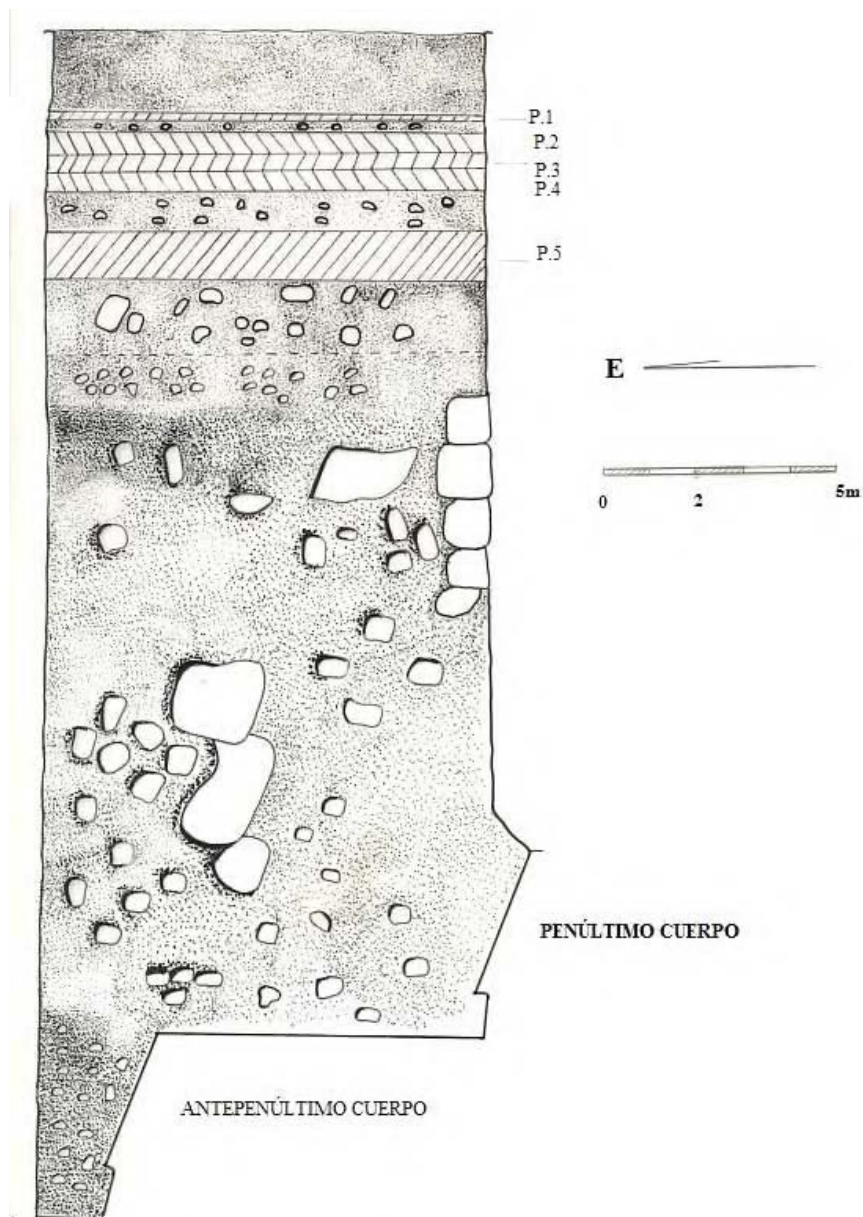
Figura 13. Edificio B-sub 1, estratigrafía.
