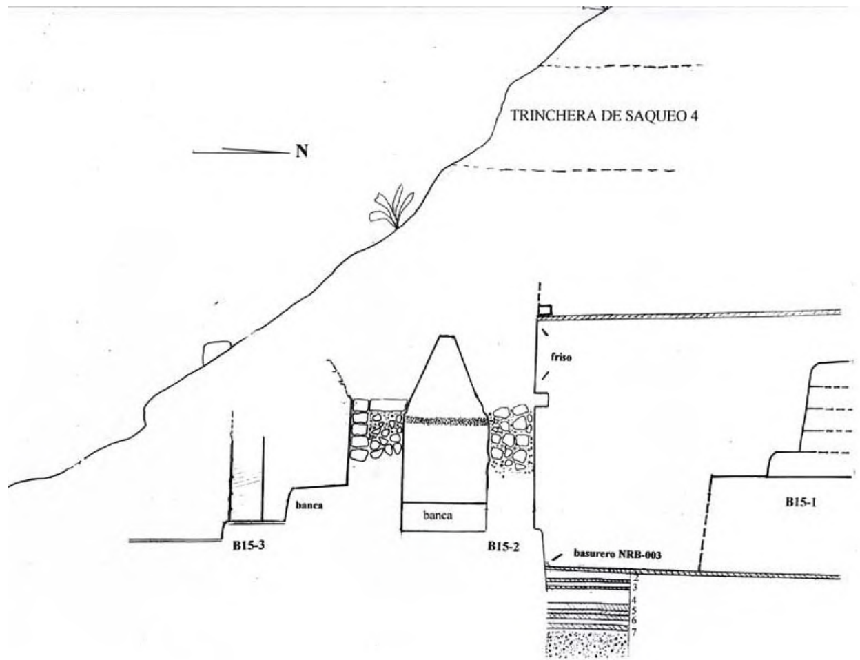
Figura 23. Subestructuras de Palacio B-15, primer nivel.
