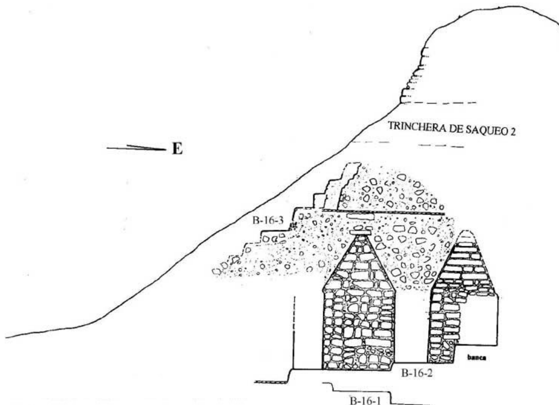
Figura 28. Palacio B-16. Subestructuras.
