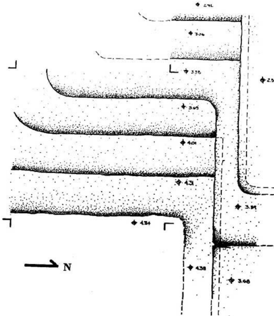
Figura 12. Subestructura B-sub 1. Detalle de planta.
