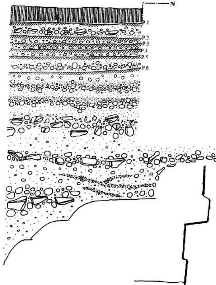
Figura 10. Suboperación E-10. Lado Oeste.
