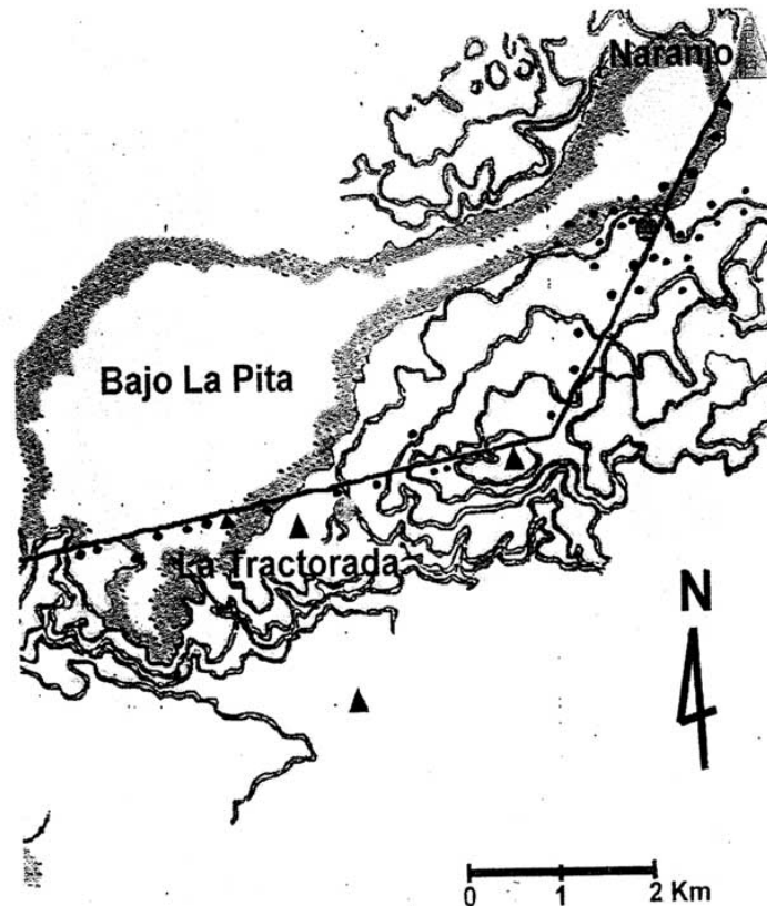
Figura 3. Transecto Yaxhá-Naranjo
